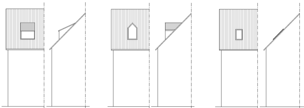
lucarne à 1 pan (« chien assis »)
